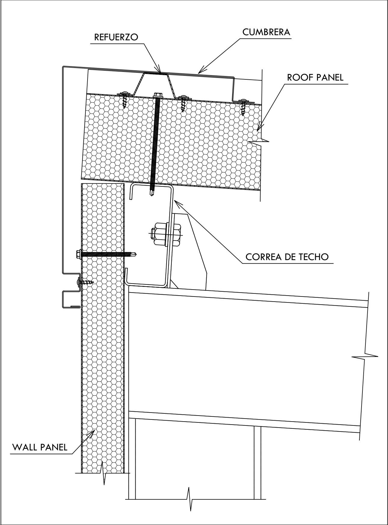
Detalle 1/2 Cumbre.
