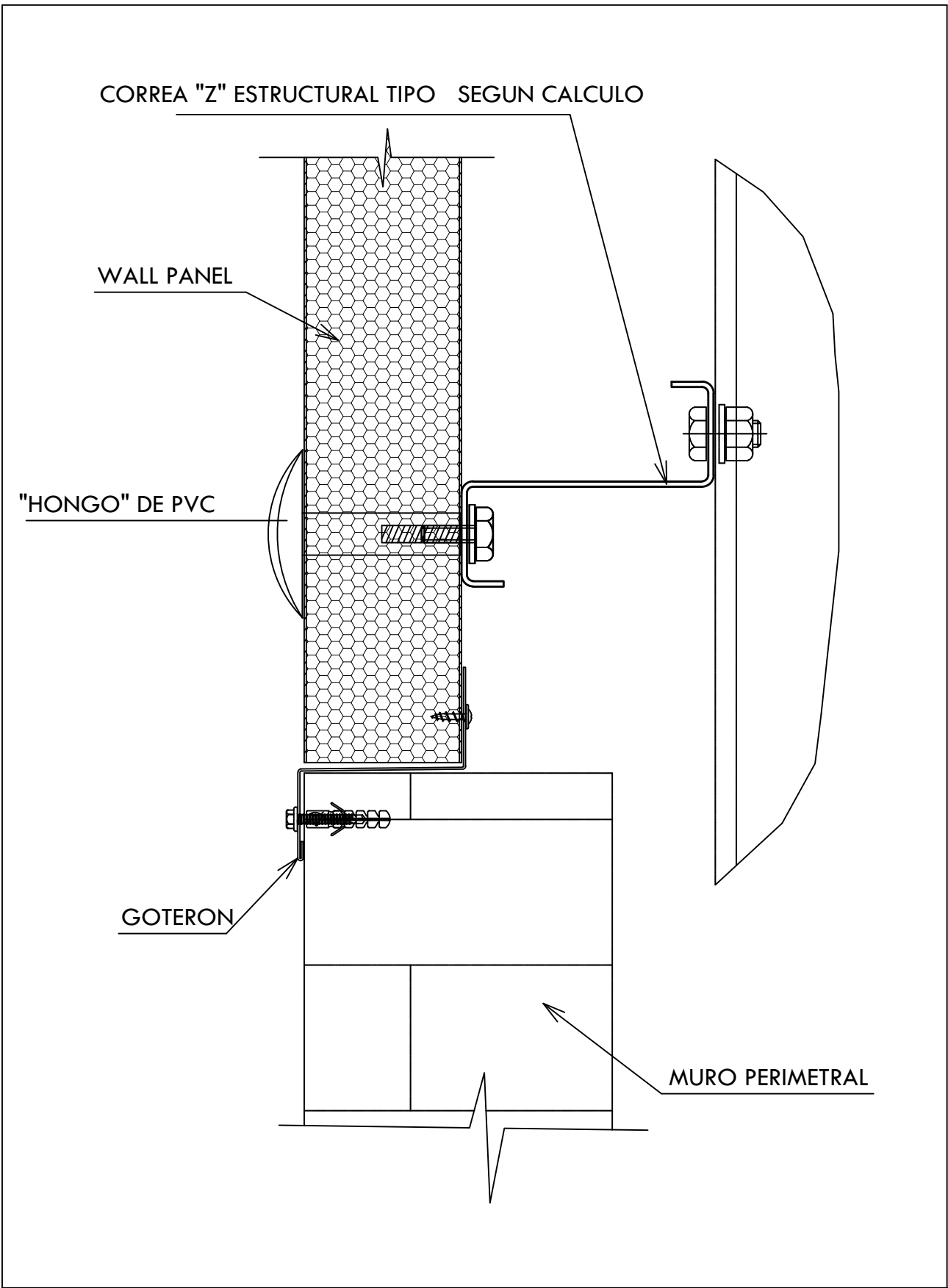
Fijacion por medio de "Hongo" de pvc.
