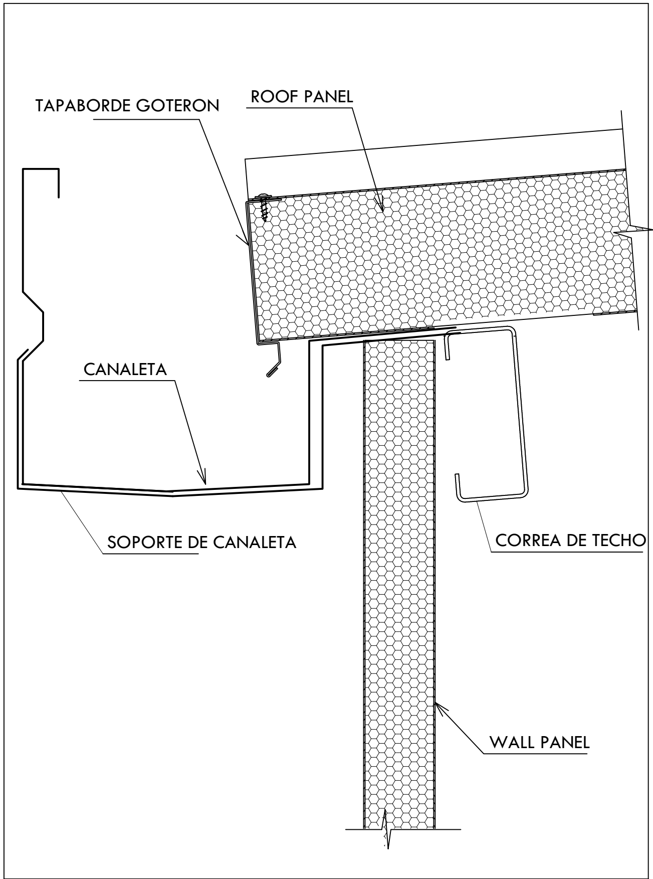
Canaleta pluvial y tapaborde de frente.
